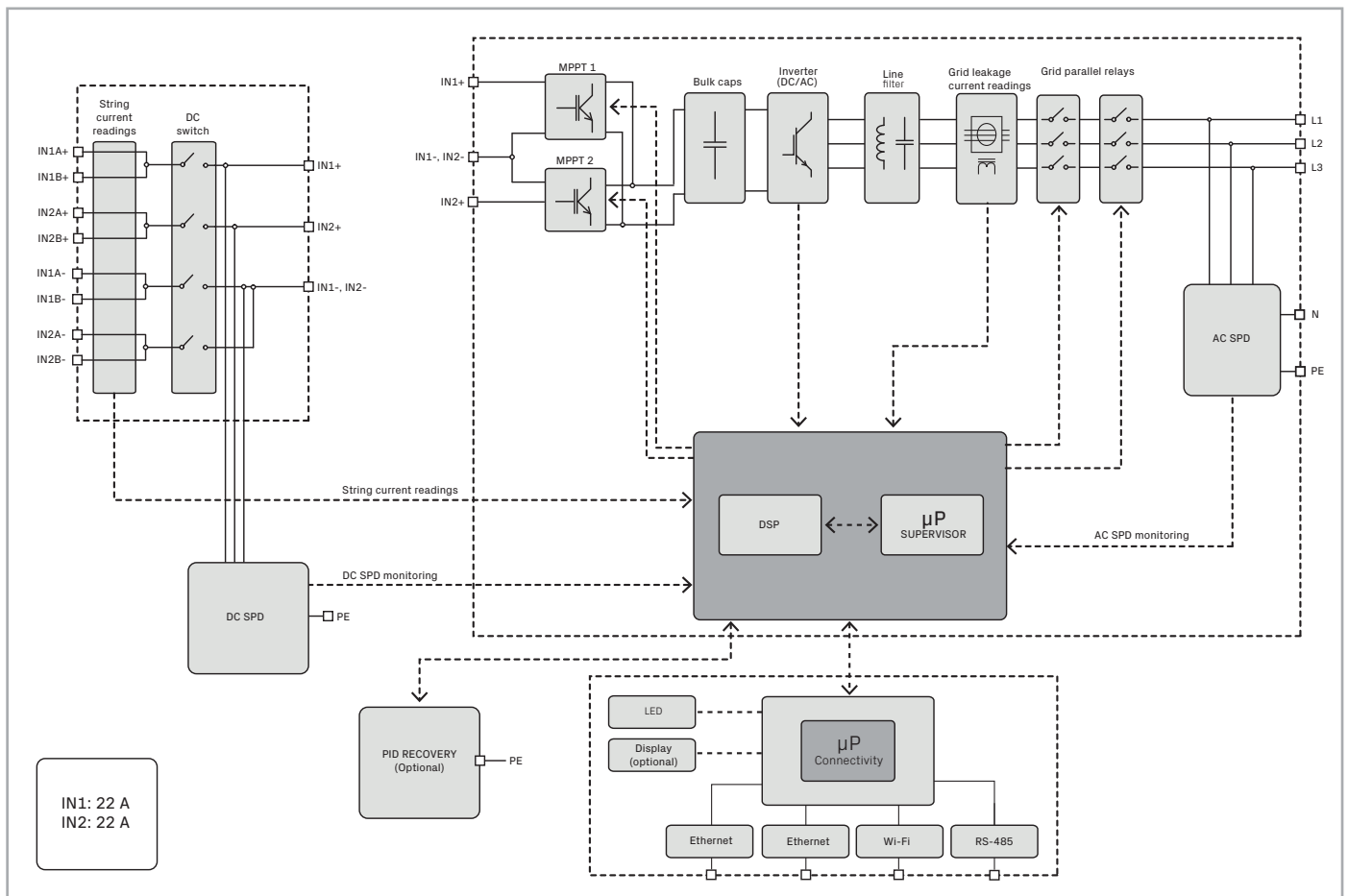
Blockschaltbild PVS-10-12,5-15-TL
